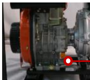
Заливная пробка с масляным щупом
