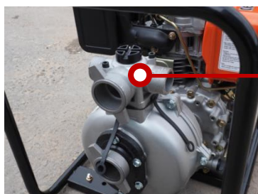
Заливная горловина. Перед первым пуском достаточно залить воду в корпус мотопомпы, воздух во всасывающем шланге она прокачает сама.
