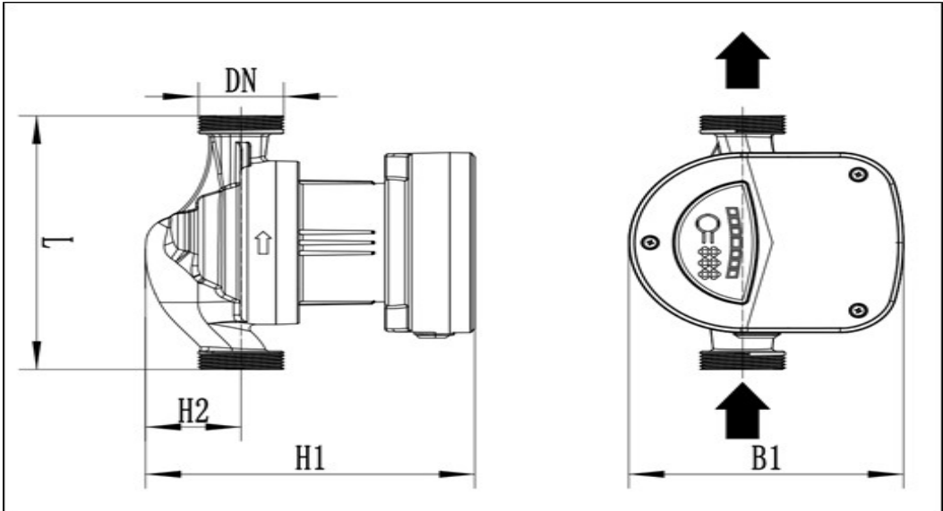
Размеры, мм
