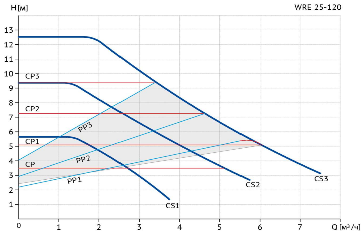
Диаграмма характеристик
