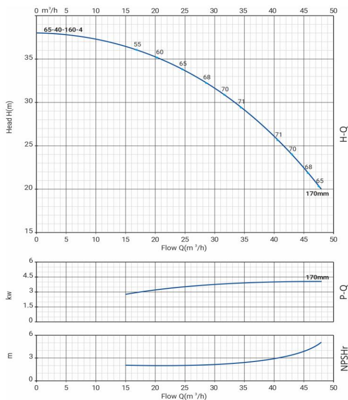
Диаграмма характеристик
