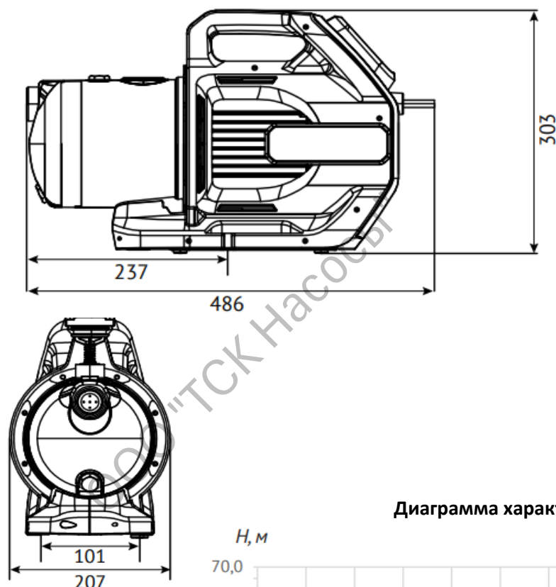
Габаритный чертёж
