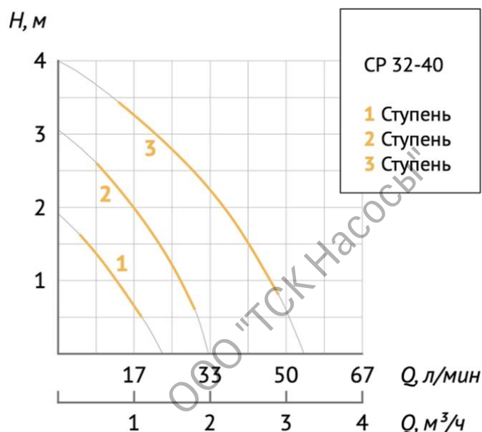
Диаграмма характеристик
