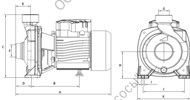
Габаритный чертёж
