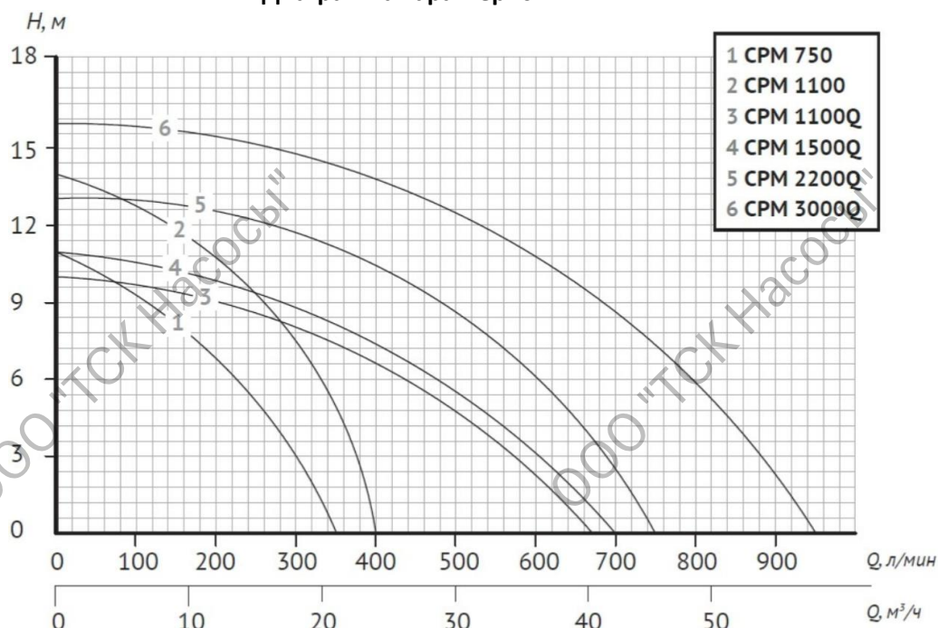
Диаграмма характеристики
