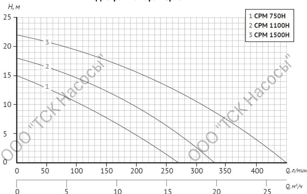
Диаграмма характеристики
