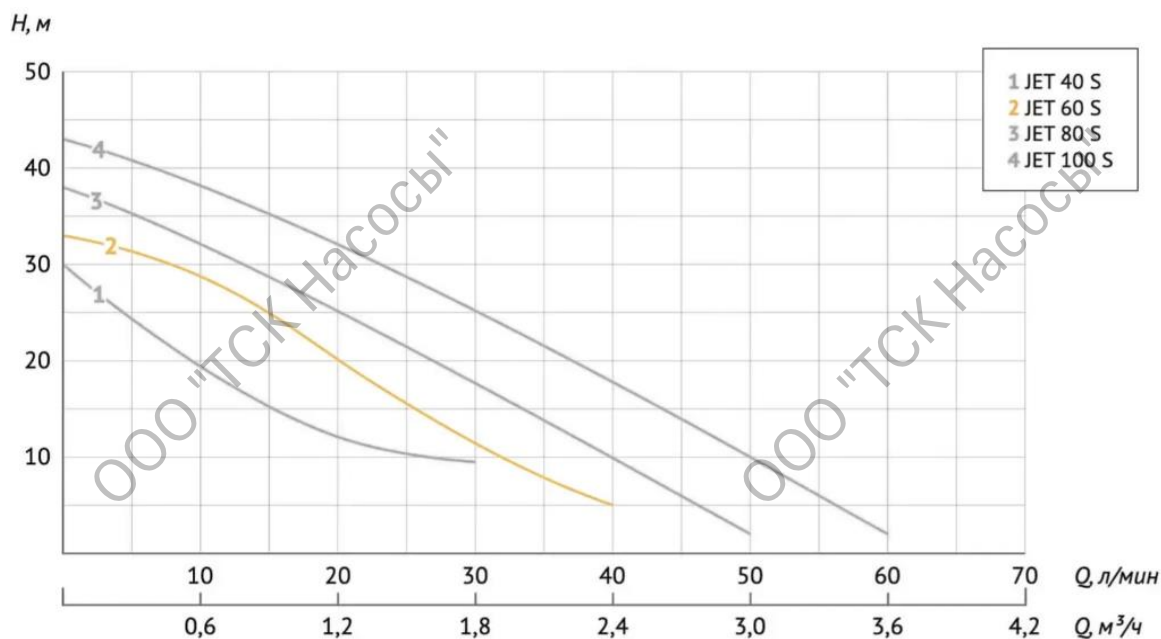
Диаграмма характеристики
