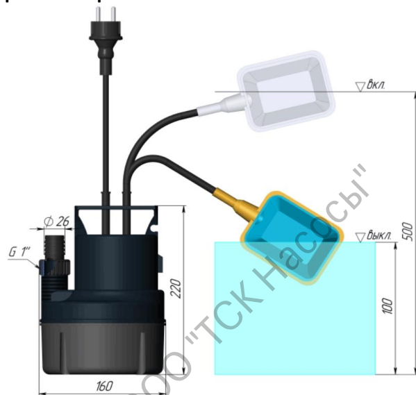
Габаритный чертёж
