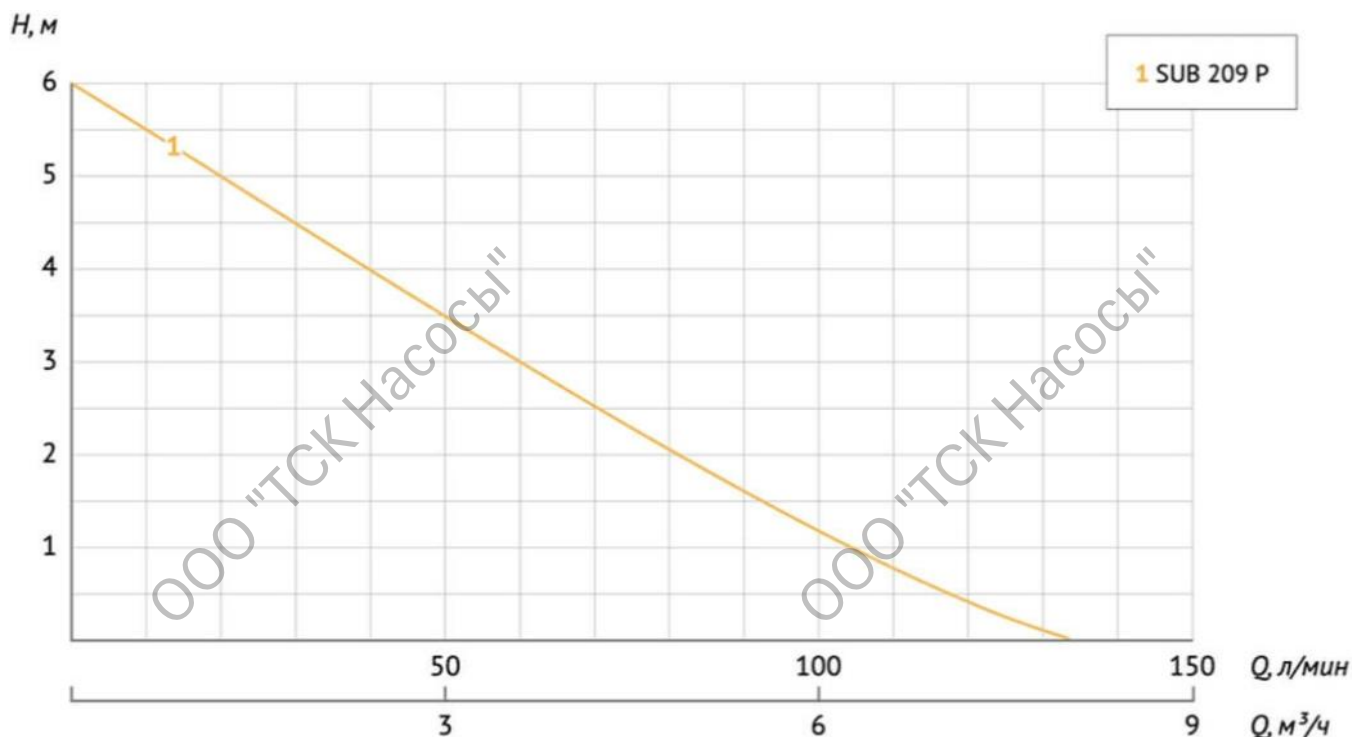
Диаграмма характеристик
