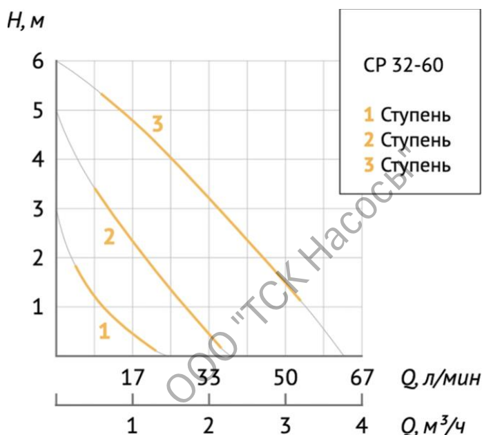
Диаграмма характеристик
