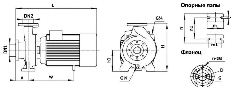
Габаритный чертеж
