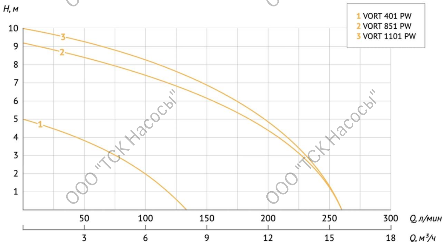
Диаграмма характеристик
