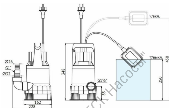
Габаритный чертёж
