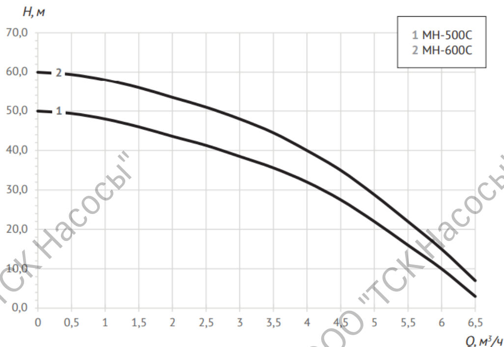
Диаграмма характеристики
