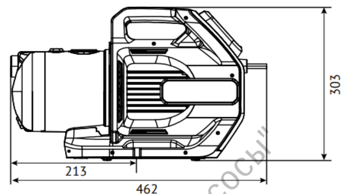
Габаритный чертёж
