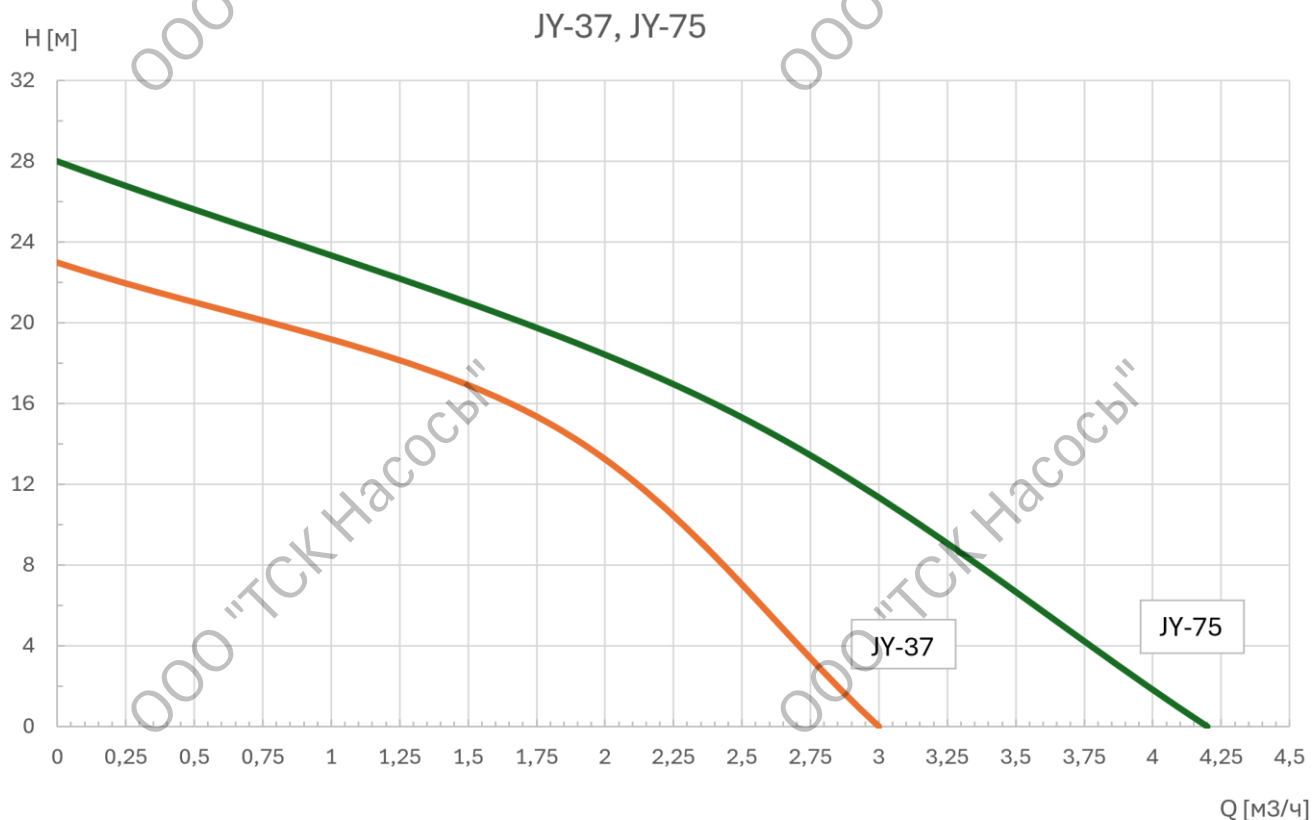
Диаграмма характеристик
