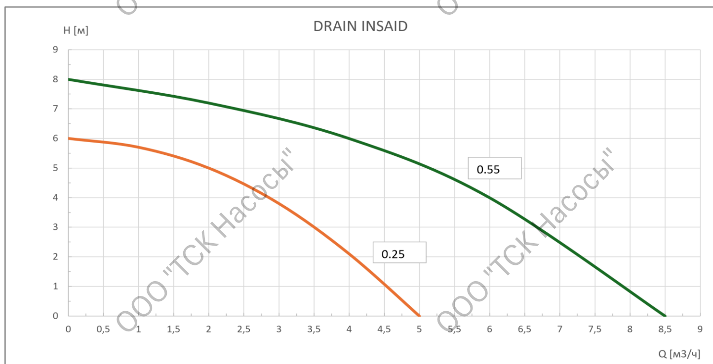
Диаграмма характеристик
