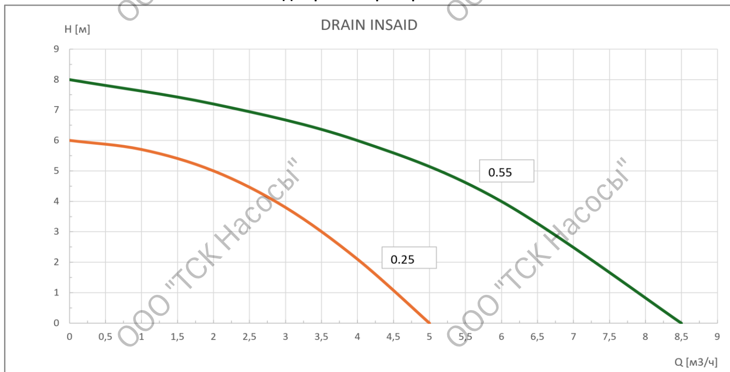
Диаграмма характеристик
