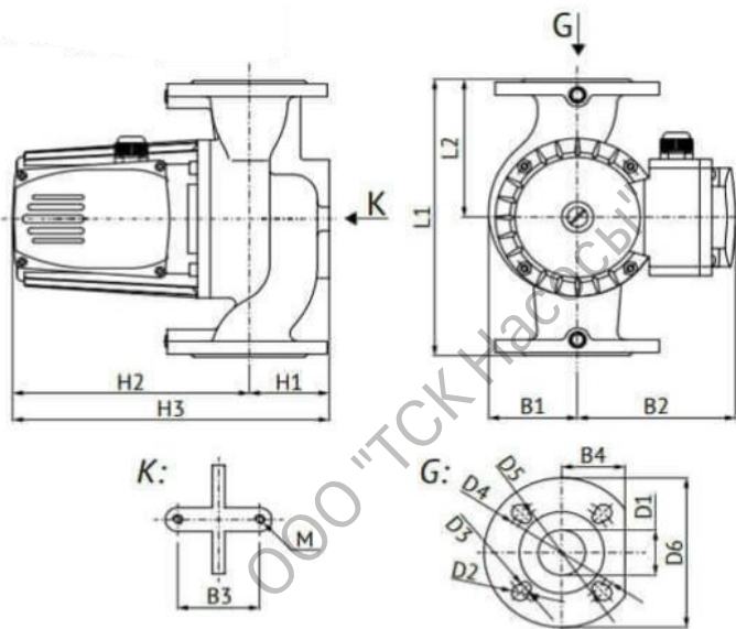
Габаритный чертёж
