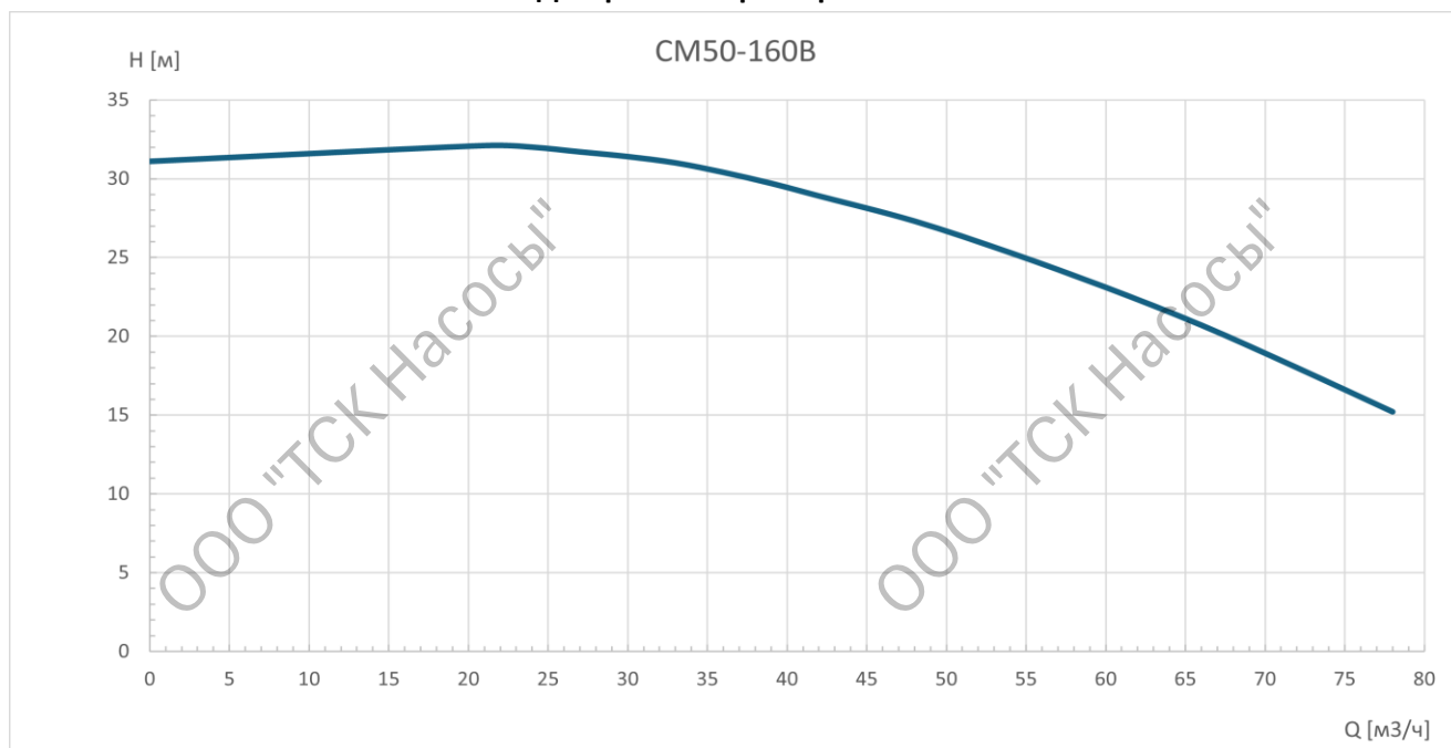
Диаграмма характеристик
