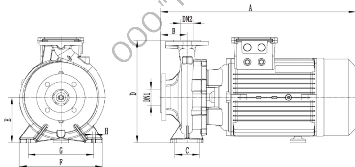
Габаритный чертёж
