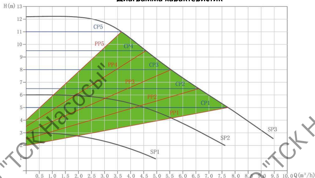
Диаграмма характеристик
