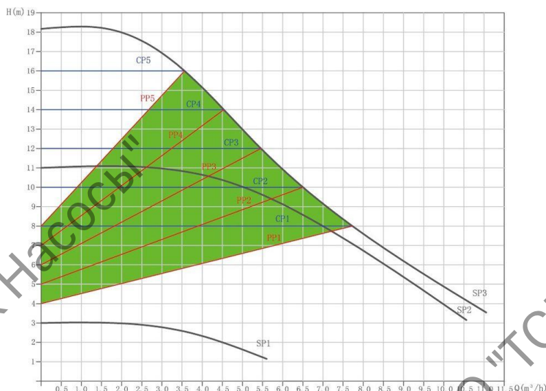
Диаграмма характеристик
